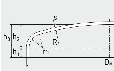
COUVERCLE
