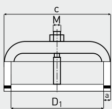
TROUS D'INSPECTION ET TROUS D'HOMME AVEC DE COUVERCLES PLAT USINÉ
