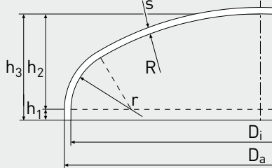
FOND ELLIPTIQUE
