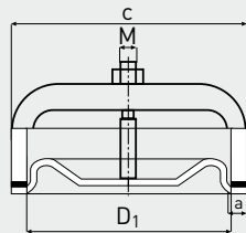
TROUS D'INSPECTION ET TROUS D'HOMME AVEC DES COUVERCLES EMBOUTIS
