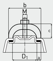
TROUS D'INSPECTION ET TROUS D'HOMME AVEC DES COUVERCLES EMBOUTIS
