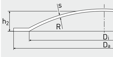
COUVERCLE
