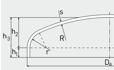
CALOTTE SPHÉRIQUE
