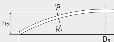
DIFFUSEURBODEN
