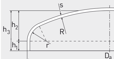
GEWÖLBTE SCHEIBE
