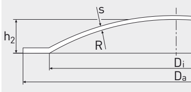
TELLERBODEN
