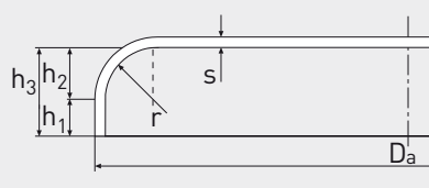
ELLIPTISCHER BODEN
