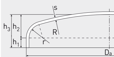
NORMAL-/FLACHGEWÖLBTER BODEN
