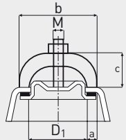
SCHAU- UND HANDLOCH- VERSCHLÜSSE
