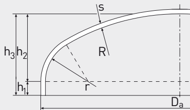
KORBBOGENBODEN
