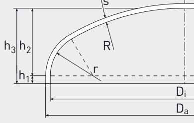
ELLIPTISCHER BODEN
