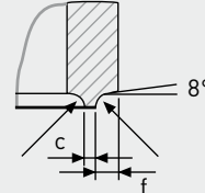
FORM DU DOUBLE U
